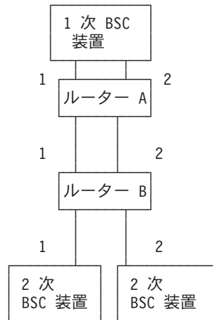
図31. バーチャル BSC リレー・マルチポイント構成. 図の中の数字は、BSC リレーのグループ番号を表しています。
