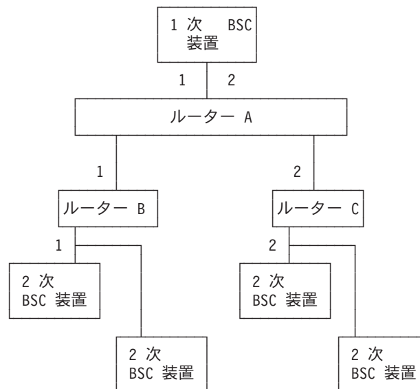
図32. バーチャルおよび物理 BRLY マルチポイント構成の組み合わせ. 図の中の数字は、BSC リレーのグループ番号を表しています。
